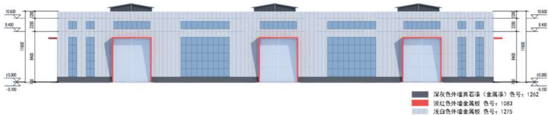
A-K立面图
