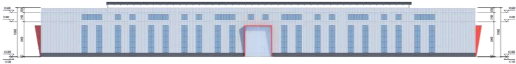
A-K立面图
